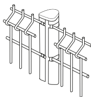
Unión de verja en plano
