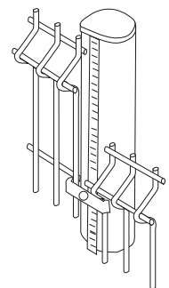
Unión de verja en desniveles
